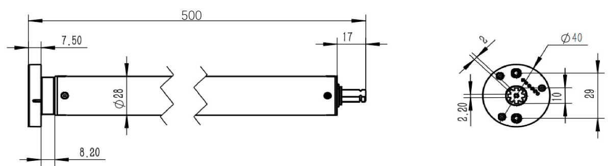
产品尺寸 (mm)
