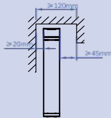
单轨电动窗帘 窗帘盒预留最小尺寸
