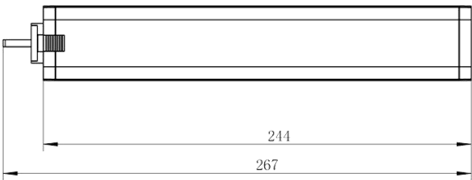
产品尺寸 (mm)
