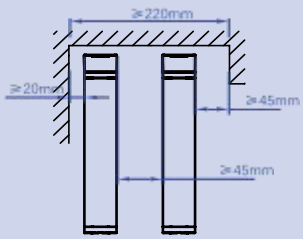
双轨电动窗帘 窗帘盒预留最小尺寸
