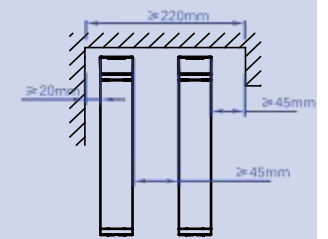
双轨电动窗帘 窗帘盒预留最小尺寸
