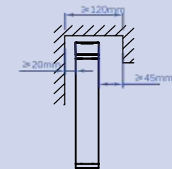
单轨电动窗帘 窗帘盒预留最小尺寸
